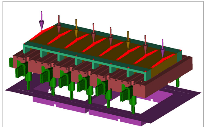
100-ton press die bolster model
